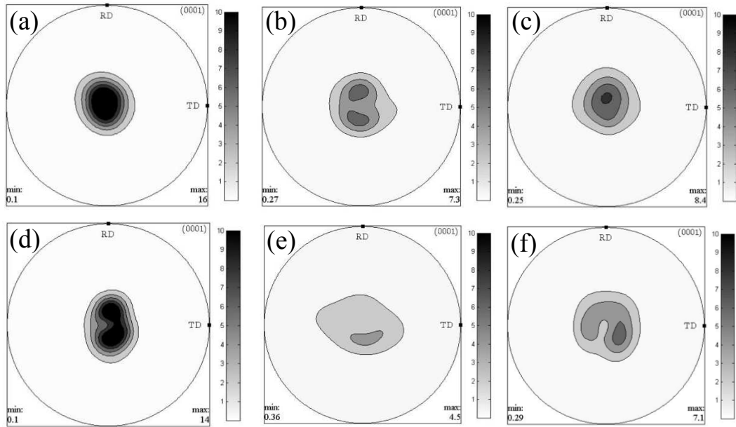
FIGURE 1. Basal pole figures for (a) Mg-0.009at.% Y (b) Mg-0.15at.% Y (c) Mg-0.024at.% Nd (all as rolled) (d) Mg-0.009at.% Y (e) Mg-0.15at.% Y (f) Mg-0.024at.% Nd (after annealing for 1h at 673 K (400 Celsius)).
