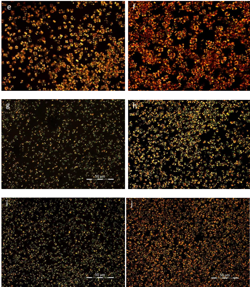
Figure 9. PLOM photos of a) PEF at 160°C, 10 min, b) PEF at 180°C, 15 min, c) PEF at 200°C, 20 min, d) PEF at 210°C, 30 min, e) PEFSu 92/8 at 150°C, 20 min, f) PEFSu 92/8 at 160°C, 20 min, g) PEFSu 87/13 at 140°C, 20 min, h) PEFSu 87/13 at 160°C, 20 min, i) PEFSu 81/19 at 130°C, 20 min and j) PEFSu 81/19 at 140°C, 20 min.
